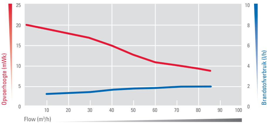
Prestaties van de PAV3-85
